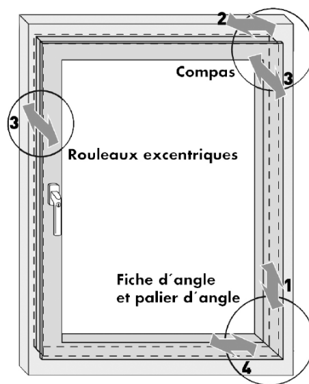
4. Réglage latéral bas
