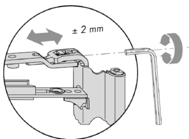
3. Réglage de la pression de l'ouvrant sur le dormant
