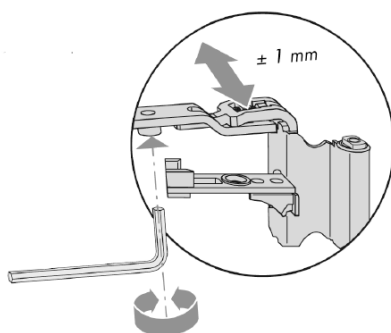
3. Réglage de la pression de l'ouvrant sur le dormant
