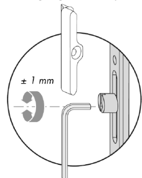
3. Réglage de la pression de l'ouvrant sur le dormant
