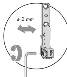
4. Réglage latéral bas
